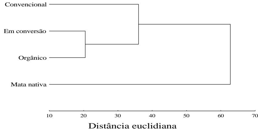
Figura 2 - Dendrograma de dissimilaridade entre o fragmento de mata nativa e os sistemas de produção do cafeeiro: convencional, em conversão e orgânico, em função das variáveis de física do solo na profundidade de 0-20 cm.
