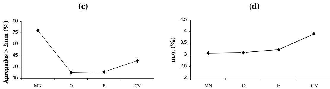
Figura 1 - Alterações nas características físicas de um LE, sob mata nativa {MN} e cultivado com cafeeiros em sistemas de produção convencional {CV}, em conversão {E} e orgânico{O}.
