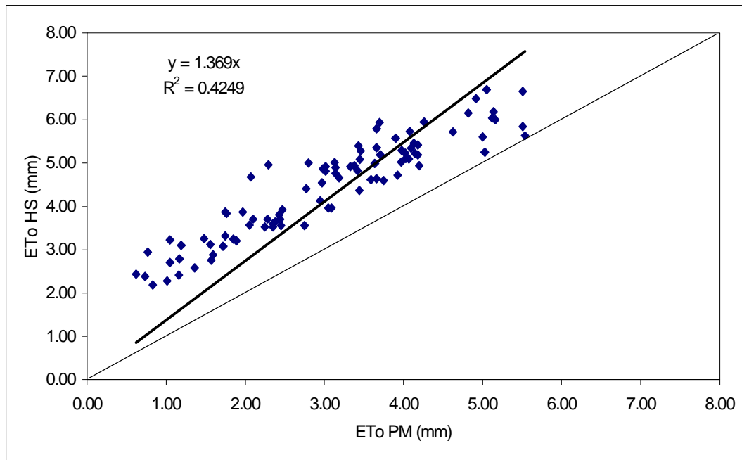
Figura 2 - Valores diários de ETo estimados pelos métodos de Penman-Monteith (PM) em relação ao método de Hargreaves e Samani (HS), gerados pelo software SISDA, e a equação de regressão linear forçada pela origem.
