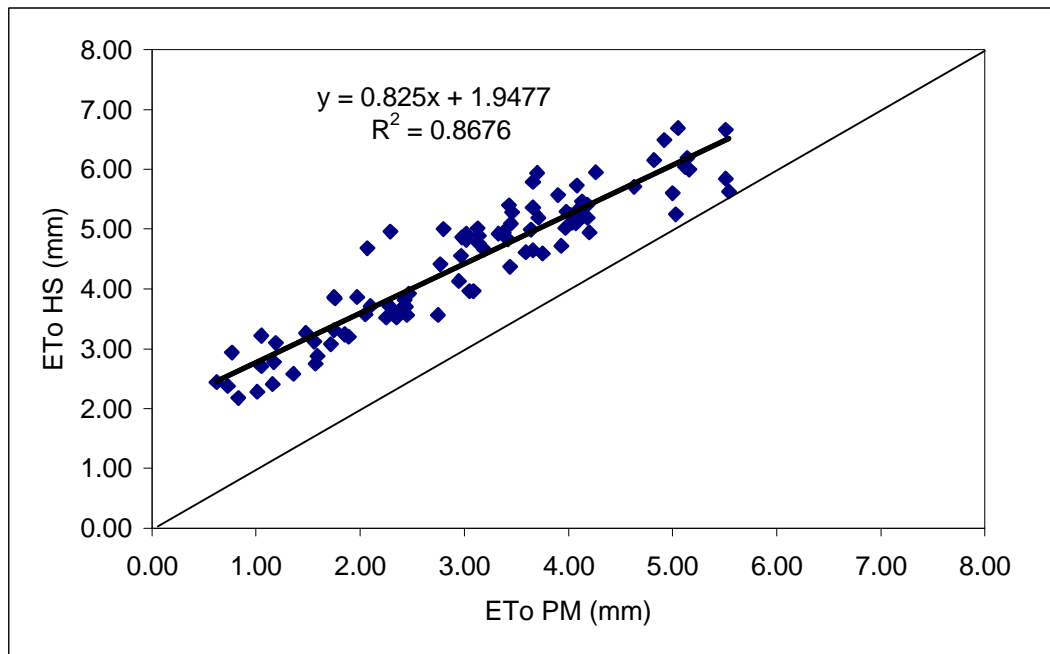
Figura 1 - Valores diários de ETo estimados pelos métodos de Penman-Monteith (PM) em relação ao método de Hargreaves e Samani (HS), gerados pelo software SISDA, e a equação de regressão linear completa.
